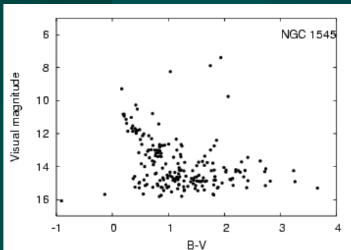
球状星団NGC1545のHR図 (2006年度卒業研究より)
