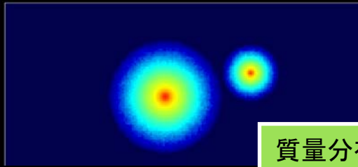
銀河団衝突のシミュレーション
